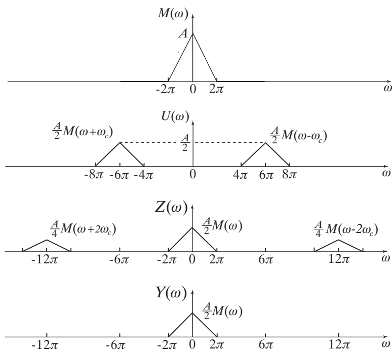
Σχήμα 5.1 Τα φάσματα της άσκησης για \omega_c = 6\pi .
