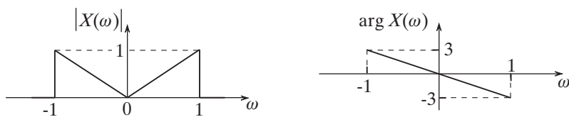
Σχήμα 4.1 Το μέτρο και η φάση του MF του σήματος
